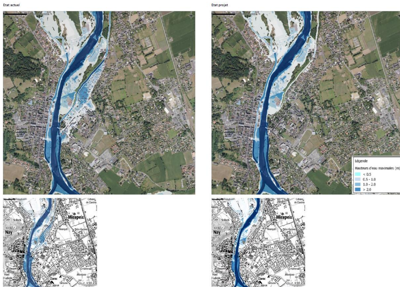
Figure 35: Zone d'influence hydraulique du mur anti-crue
