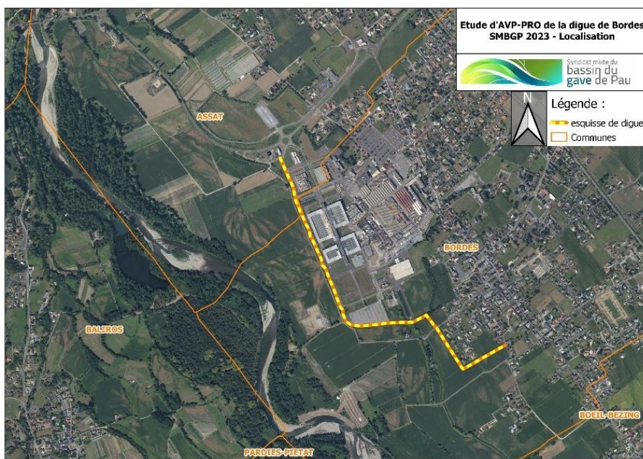
Figure 24: Implantation de la digue de Bordes
