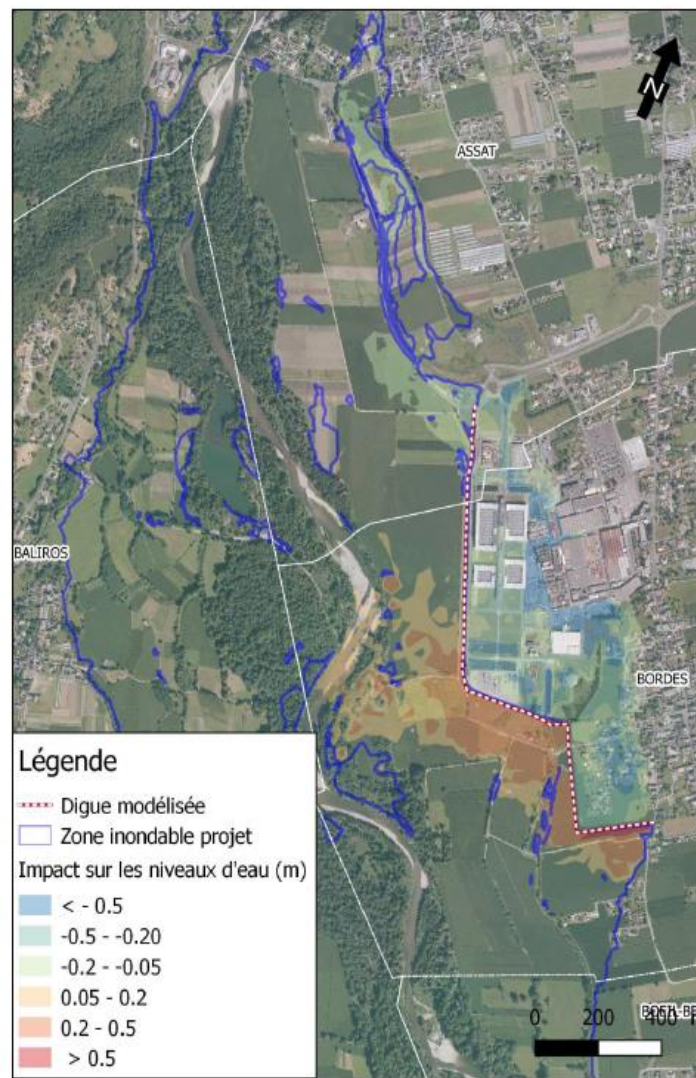
Figure 26: impacts hydrauliques de la digue de Bordes
