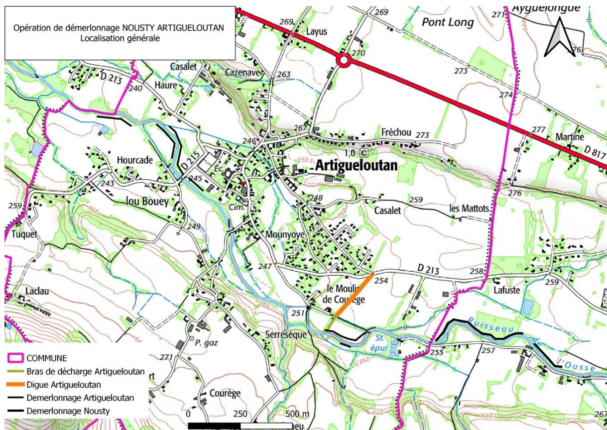
Figure 43: Projet de démerlonnage du les communes de Nousty et Artigueloutan
