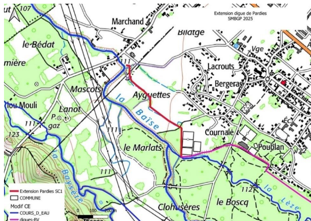
Figure 28: Réfection et prolongement de la digue de Pardies
