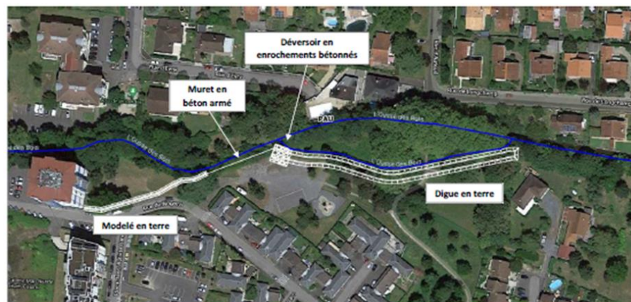
Figure 27 : réfection de la digue du quartier Nogaro
