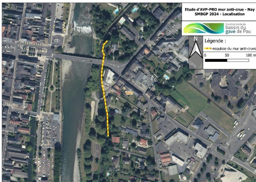
Figure 33: Implantation du mur anti-crue de Nay
