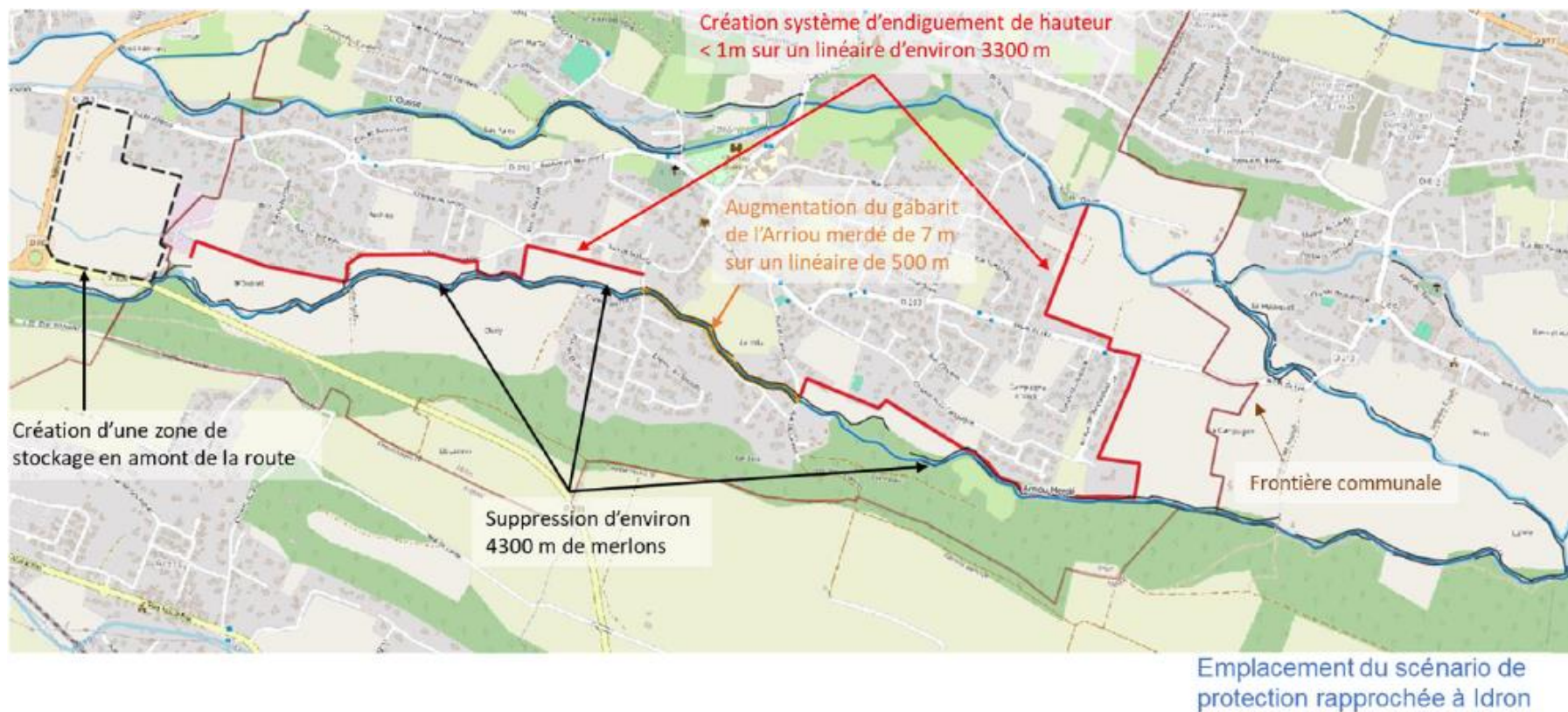
Figure 32: Schéma du système de protection rapprochée à Idron
