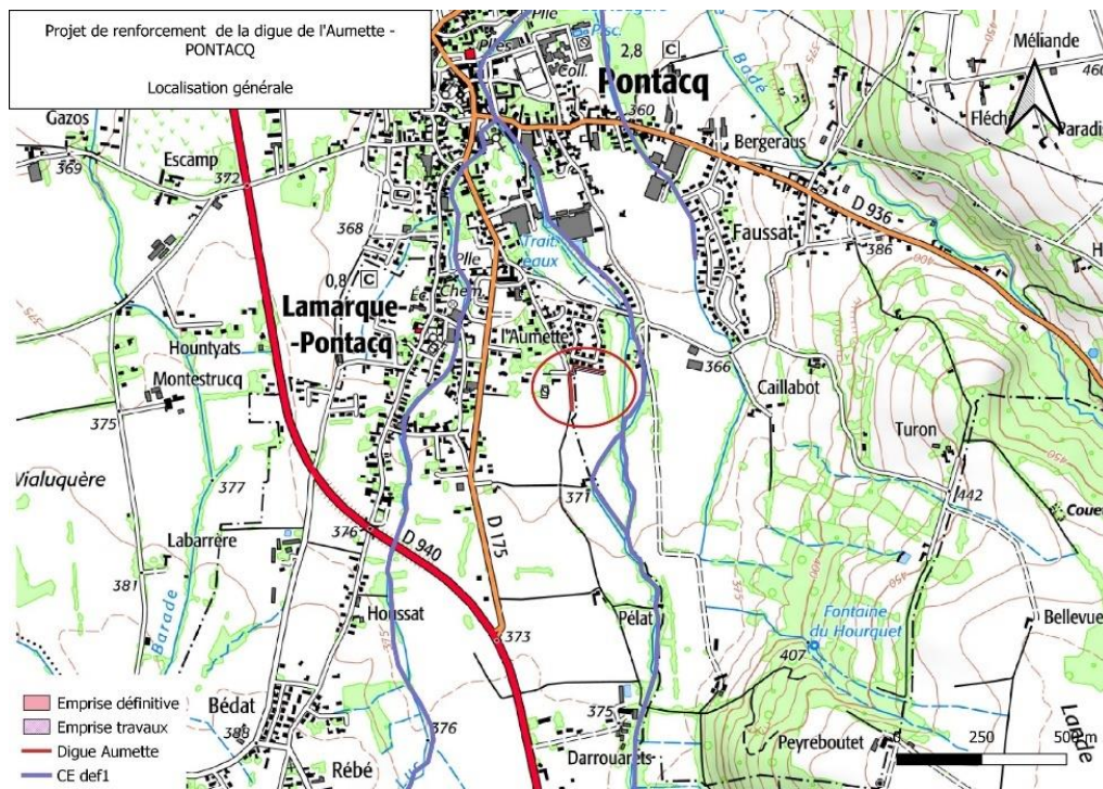
Figure 29: Réfection de la digue de l'Aumette à Pontacq
